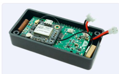
balise GPS LoRa Matériel et logiciel libres et ouverts
