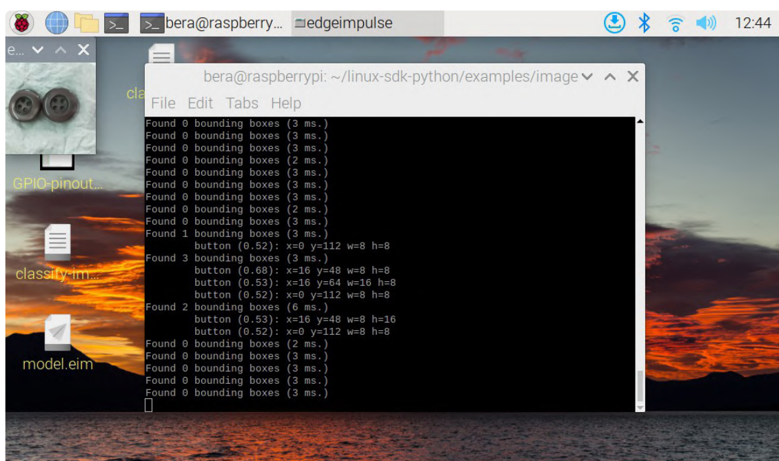
Figure 7. Après avoir retiré un bouton, le modèle l'a compté correctement du premier coup.
